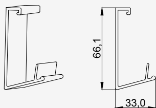
Klipsz
