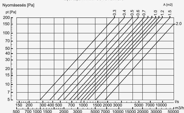
120Z lamella nyomásesés 120mm-es kiosztással 2,5x2,5x1mm-es rovarháló
